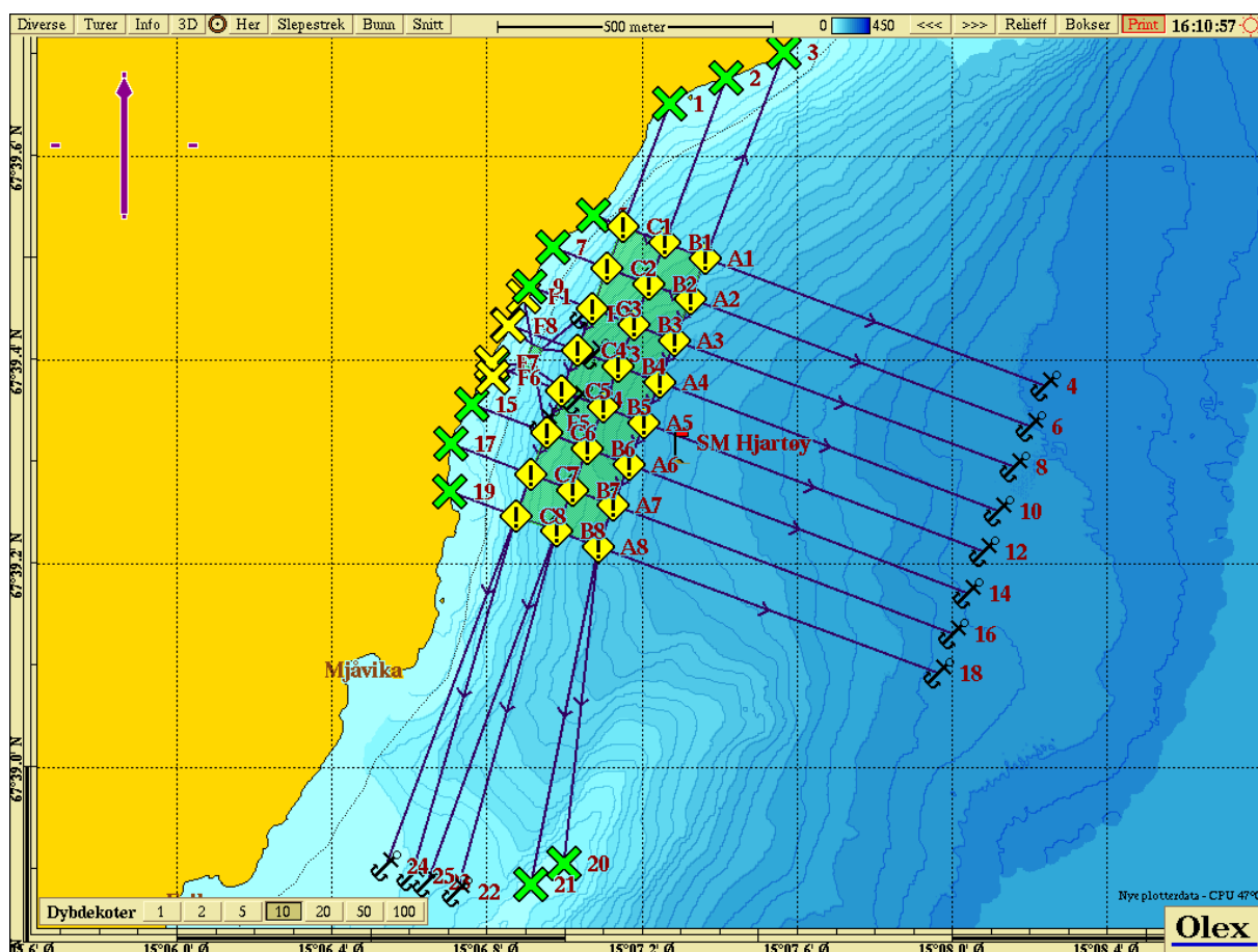
Figur 1. Plassering av strømmålerrigg i forhold til lokaliteten Hjørtøy Ø.
