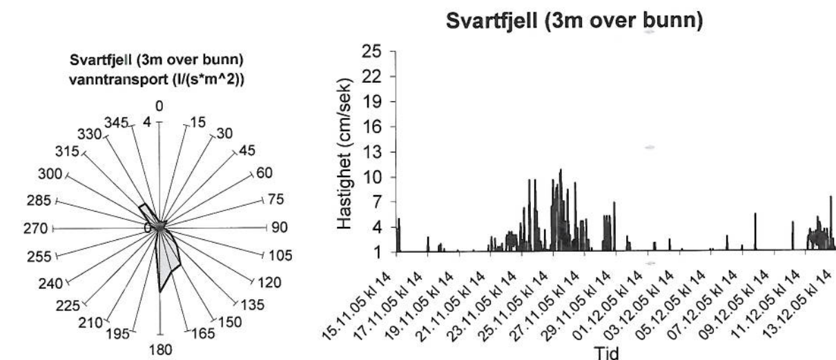
Figur 31. Strømretninger, vanntransport og strømhastighet på lokalitet Svartfjell 15.11. – 13.12. 05. 3 meter over bunn ved 112 meters bunndyp.
