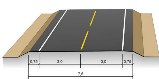
Figur 4. Tverrprofil for Hø2 (mål i m)
