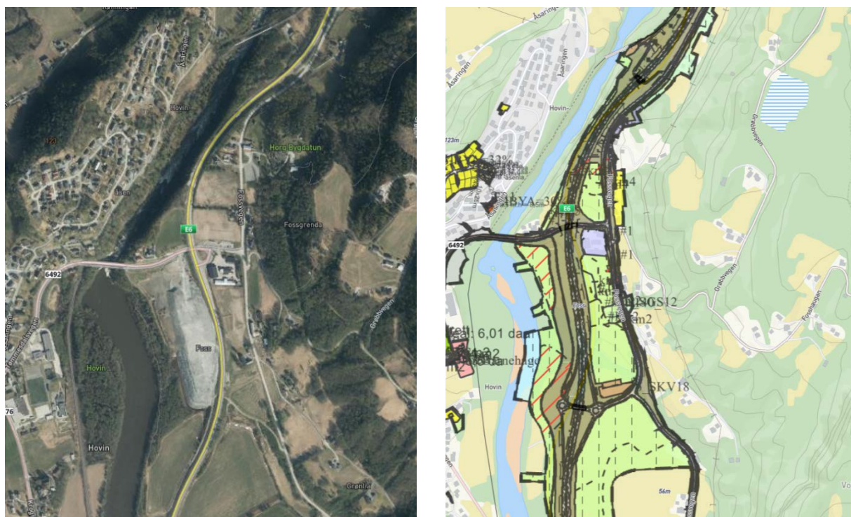
Figur 6 - I området ved avkjøring til Hovin er det i gjeldende plan regulert et toplans kryss. I optimaliseringen vil en forbedret trafikal løsning vurderes, samtidig som det er et mål at kryssutforming skal gi redusert massebehov samt mindre beslag av permanent og midlertidig jordbruksareal.
