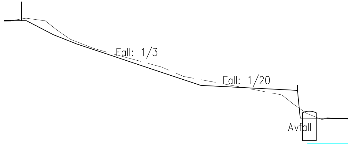
SNITT B-B
